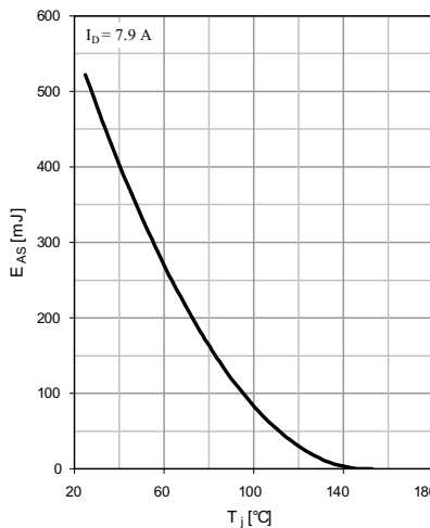
Fig. 10 Avalanche energy
