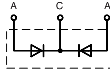
TO-263 AB
