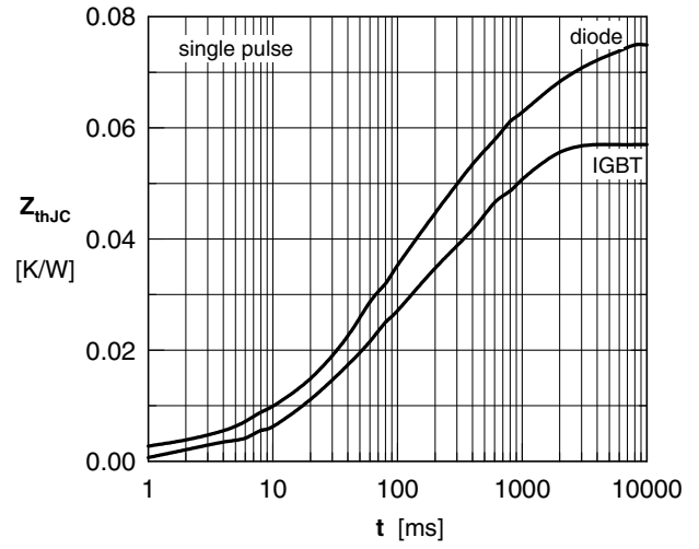
Fig. 8 Typ. transient thermal impedance
