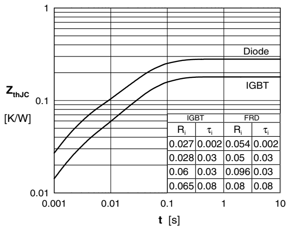
Fig. 9 Typ. transient thermal impedance
