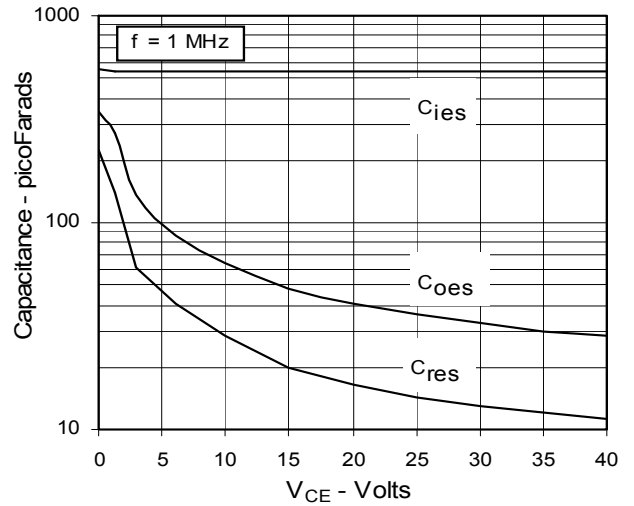
Fig. 16. Capacitance
