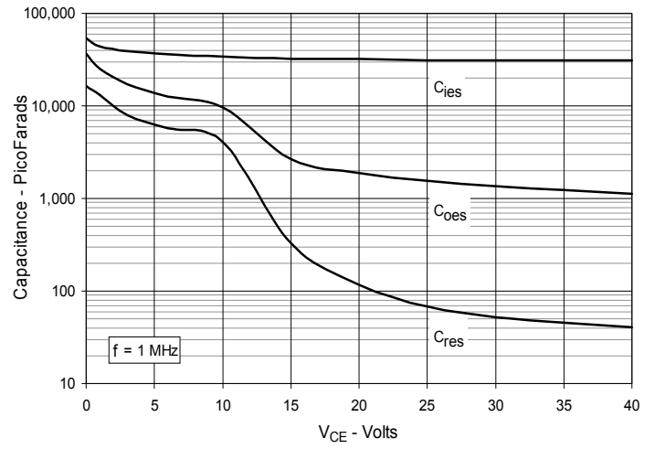
Fig. 8. Capacitance
