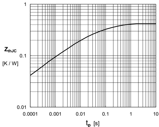
Fig. 26. Transient thermal impedance
