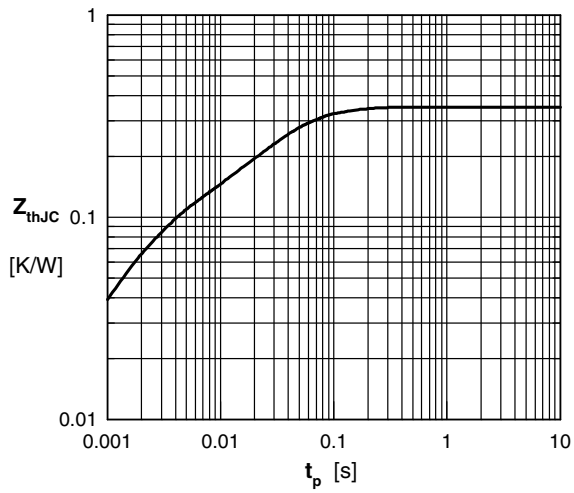
Fig. 7 Typ. transient thermal impedance
