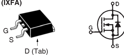
TO-263 AA (IXFA)
