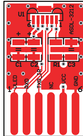
Top Layer
