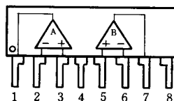
NJM4580L
