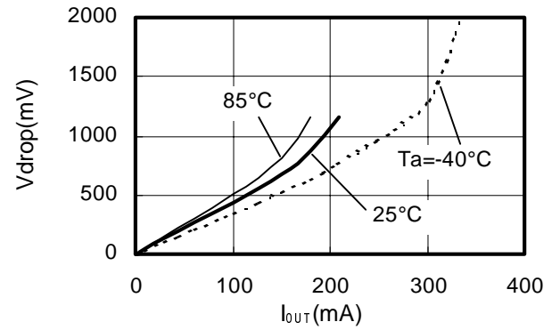
S-818A30A
