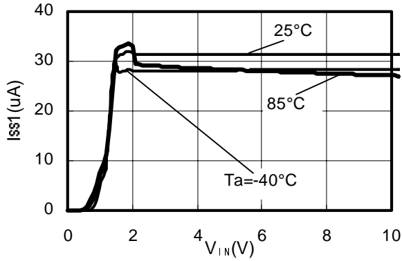
S-818A20A
