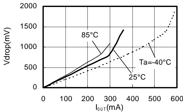
S-818A50A
