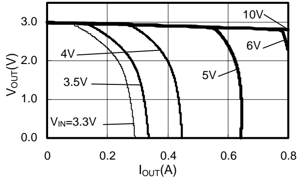
S-818A30A(Ta=25°C)
