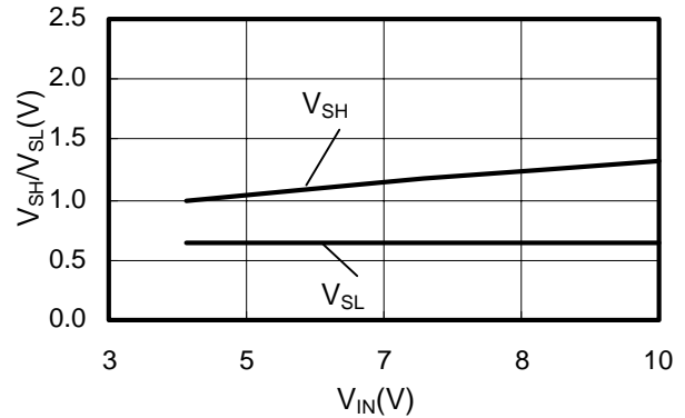
S-818A30A
