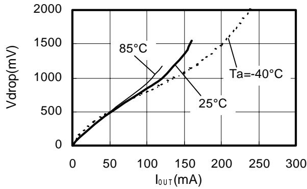
S-818A20A
