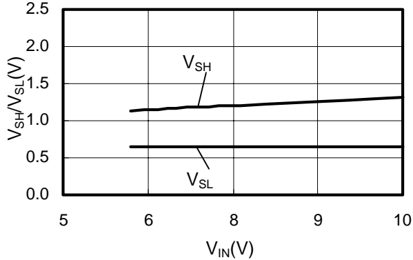
S-818A50A
