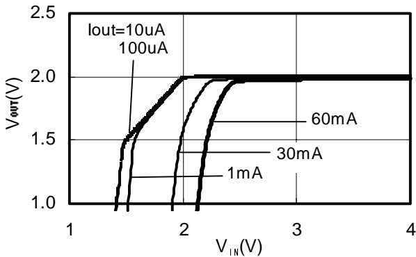
S-818A20A (Ta=25°C)
