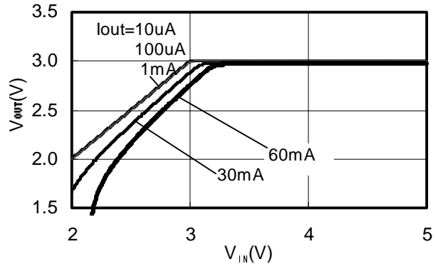
S-818A30A (Ta=25°C)
