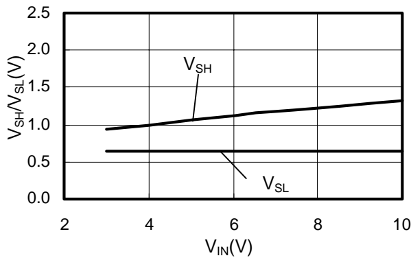
S-818A20A
