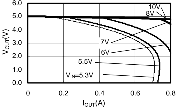
S-818A50A(Ta=25°C)
