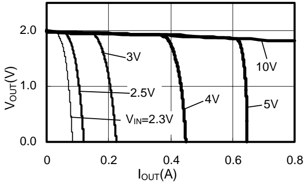
S-818A20A(Ta=25°C)
