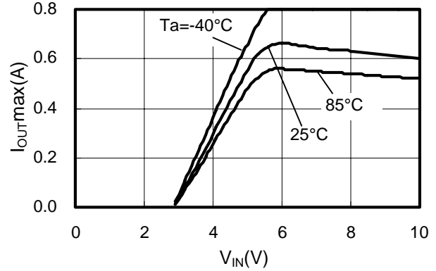
S-818A30A
