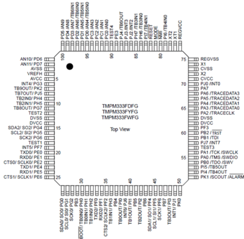
パッケージ名称 LQFP100-P-1414-0.50H
