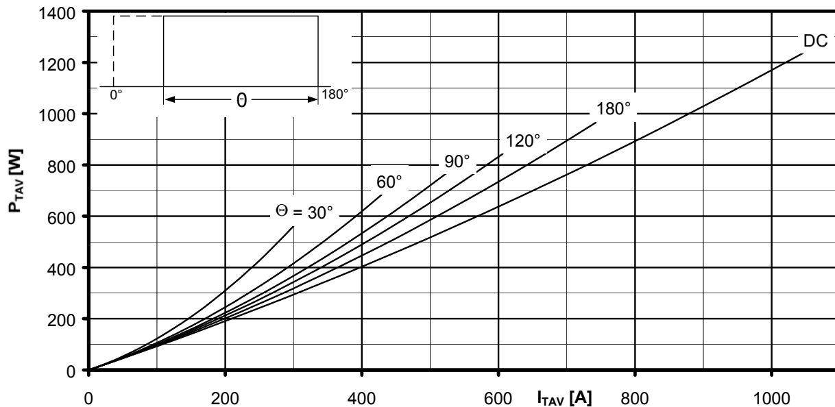
Durchlassverlustleistung je Zweig / On-state power loss per arm P_{TAV} = f(I_{TAV}) Rechteckförmiger Strom / Rectangular current Strombelastung je Zweig / Current load per arm Parameter: Stromflußwinkel / Current conduction angle \Theta
