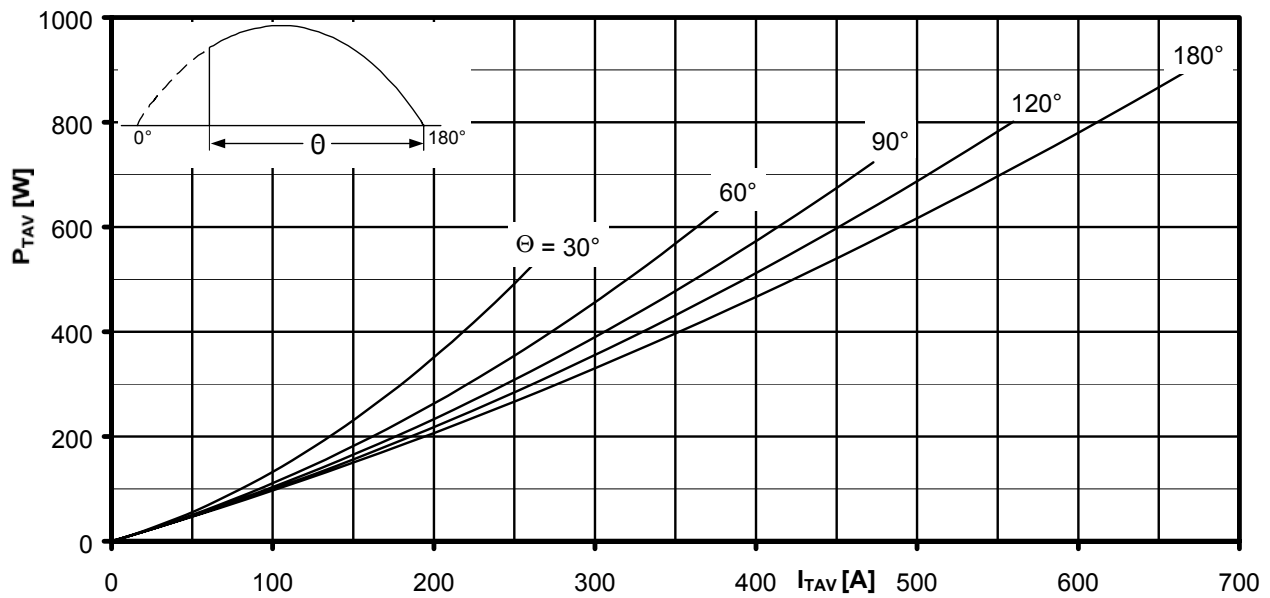
Durchlassverlustleistung je Zweig / On-state power loss per arm P_{TAV} = f(I_{TAV}) Sinusförmiger Strom / Sinusoidal current Strombelastung je Zweig / Current load per arm Parameter: Stromflußwinkel / Current conduction angle \Theta
