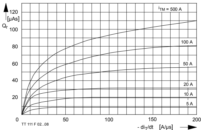
Bild / Fig. 18 Sperrverzögerungsladung Q_r = f(di/dt) t_{vj} = t_{vj} \text{ max} , v_R = 0,5 V_{RRM} , v_{RM} = 0,8 V_{RRM} Parameter: Durchlaßstrom i_{TM} / Recover charge Q_r = f(di/dt) t_{vj} = t_{vj} \text{ max} , v_R = 0,5 V_{RRM} , v_{RM} = 0,8 V_{RRM} Parameter: on-state current i_{TM}
