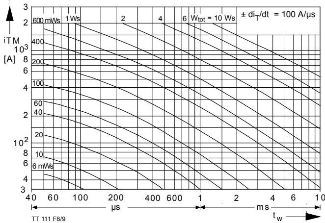
Bild / Fig. 7, 8, 9 Diagramme zur Ermittlung der Gesamtenergie W_{tot} für einen trapezförmigen Durchlaß-Strompuls, für einen Zweig bei: der angegebenen Stromsteilheit di_T/dt , Vorwärts-Sperrspannung v_{DM} \leq 0,67 V_{DRM} , Rückwärts-Sperrspannung v_{RM} \leq 50V , Spannungssteilheit dv_R/dt \leq 100 V/\mu s .
