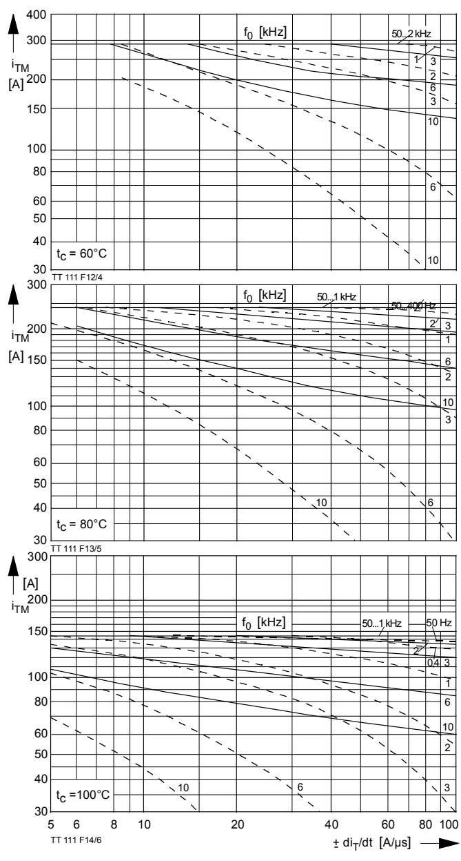
Bild / Fig. 4, 5, 6 Höchstzulässige Strombelastbarkeit in Abhängigkeit von der Stromsteilheit für ein Zweig bei: trapezförmigem Stromverlauf, der angegebenen Gehäusetemperatur t_C , Vorwärts-Sperrspannung V_{DM} \leq 0,67 V_{DRM} , Freierwendezeit t_f gemäß 5. Kennbuchstaben, Spannungssteilheit dv/dt gemäß 6. Kennbuchstaben.
