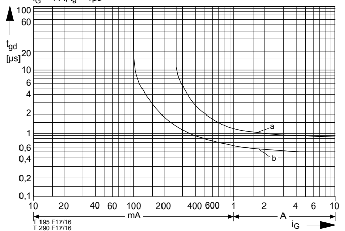
Bild / Fig. 16 Zündverzögerung/Gate controlled delay time t_{gd} , DIN 41787, t_a = 1 \mu s , t_{vj} = 25^\circ C . a - außerster Verlauf/limiting characteristic b - typischer Verlauf/typical characteristic
