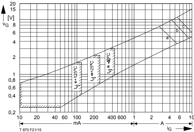
Bild / Fig. 15 Zündbereich und Spitzensteuerleistung bei v_D = 6V . Gate characteristic and peak power dissipation at v_D = 6V .
