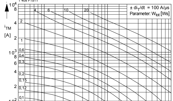
Bild / Fig. 10, 11, 12 Diagramme zur Ermittlung der Gesamtenergie W_{tot} für einen trapezförmigen Durchlaß-Strompuls, für einen Zweig bei: der angegebenen Stromsteilheit di_T/dt , Vorwärts-Sperrspannung v_{DM} \leq 0,67 V_{DRM} , Rückwärts-Sperrspannung v_{RM} \leq 0,67 V_{RRM} , Spannungssteilheit dv_R/dt \leq 600 V/\mu s .
