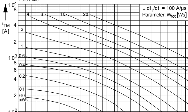
Bild / Fig. 7, 8, 9 Diagramme zur Ermittlung der Gesamtenergie W_{tot} für einen trapezförmigen Durchlaß-Strompuls, für einen Zweig bei: der angegebenen Stromsteilheit di_T/dt , Vorwärts-Sperrspannung v_{DM} \leq 0,67 V_{DRM} , Rückwärts-Sperrspannung v_{RM} \leq 50V , Spannungssteilheit dv_R/dt \leq 100 V/\mu s .
