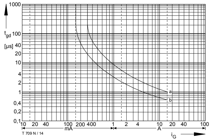
Bild / Fig. 14 Zündverzögerung / Gate controlled delay time t_{gd} = f(i_G) t_{vj} = 25 \text{ °C} , di_G/dt = i_{GM}/1\mu\text{s} a - Maximaler Verlauf / Limiting characteristic b - Typischer Verlauf / Typical characteristic
