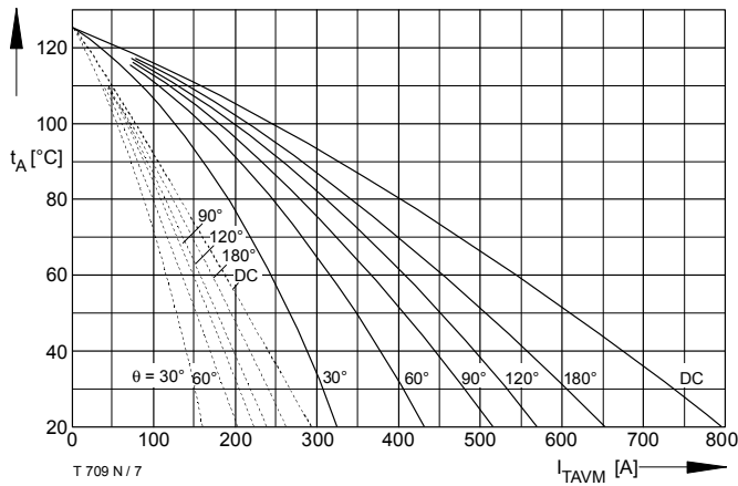
Bild / Fig. 7 Höchstzulässige Kühlmitteltemperatur / Max. allowable cooling medium temperature t_A = f(I_{TAVM}) Kühlkörper / Heatsink: K0.05F - - - - - Luftselbstkühlung / Natural air-cooling ——— Verstärkte Luftkühlung / Forced air-cooling, V_L = 30 l/s Parameter: Stromflußwinkel / Current conduction angle \theta
