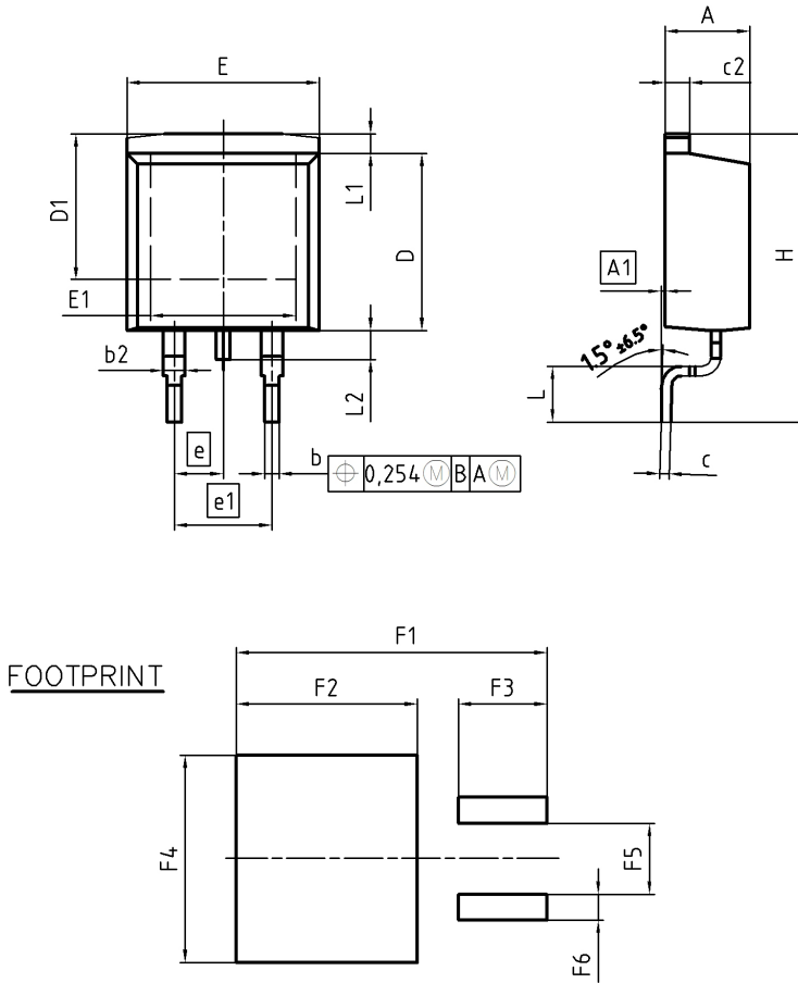
PG-TO-263-3-2
