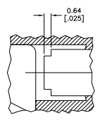
DETAIL Z SCALE: 8:1 TYP
