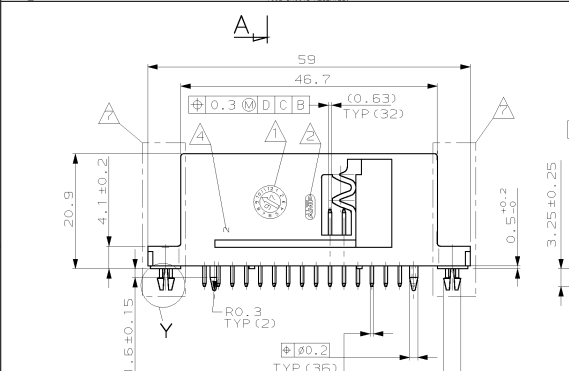
SECTION AA (COUPE)
