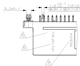
VIEW F (VUE)
