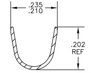
SECTION D-D
