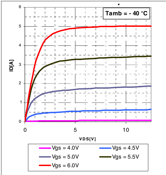
Figure 4. DC output characteristics (T amb = -40 °C)
