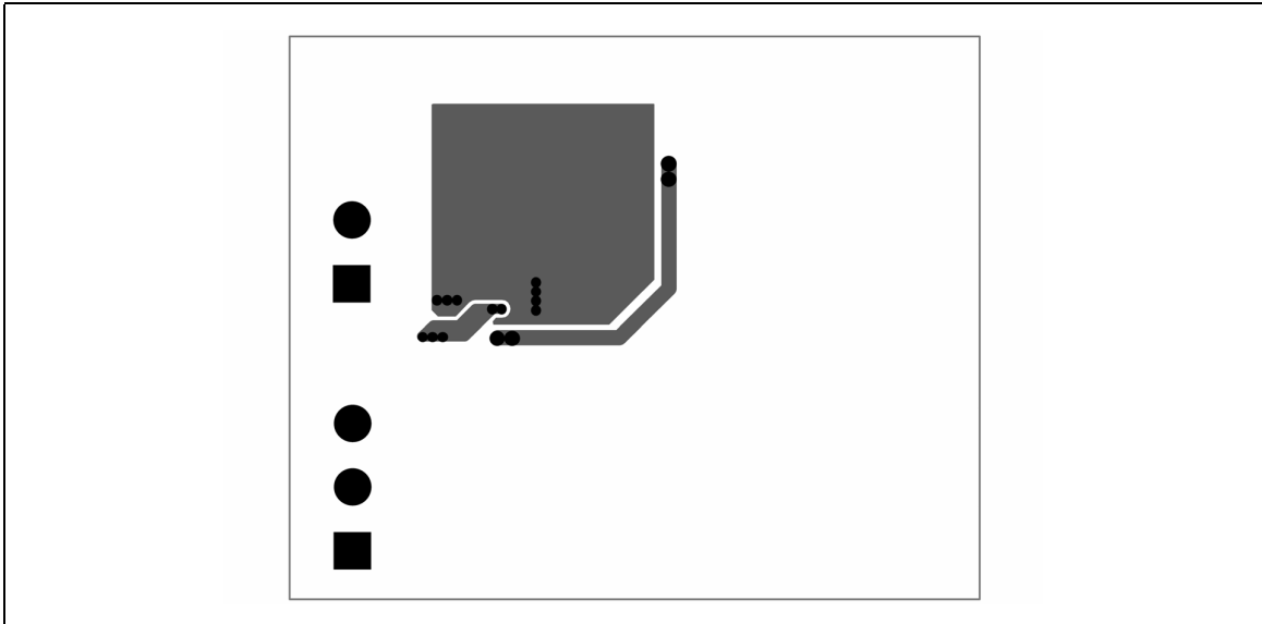
Figure 19. Bottom layer
