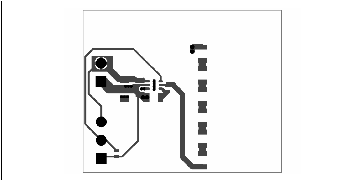
Figure 18. Top layer
