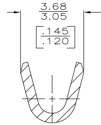
SECTION A-A SCALE 10:1
