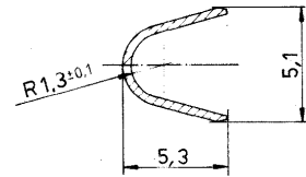
Schnitt B-B
