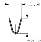
SEZIONE B-B (SECTION B-B)
