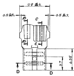
170141 - □ バラ状 LOOSE
