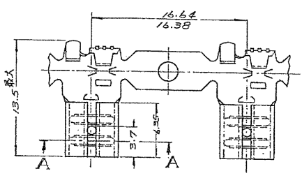
□ - 170140 - □ 連鎖状 STRIP
