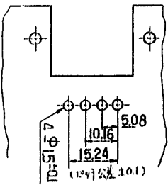
-2-3 基板加工寸法 (一般公差 ±0.15)
