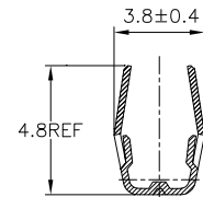
断面 B-B SECT B-B (175030のみ適用) (ONLY 175030)
