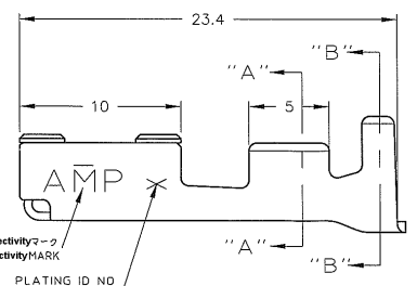
PLATING ID NO めっき ID No
