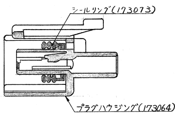
断面 A-A
