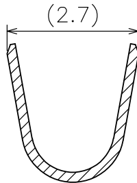
断面 B-B SECT B-B
