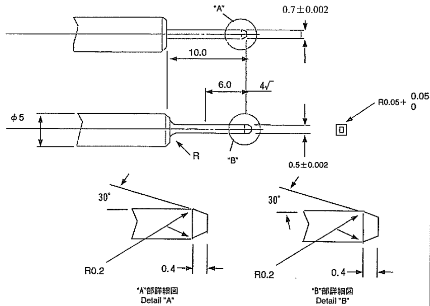
Fig. 10 コンタクト挿入引抜力測定用ゲージ
