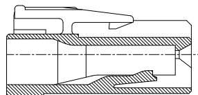
断面 A-A SECT A-A
