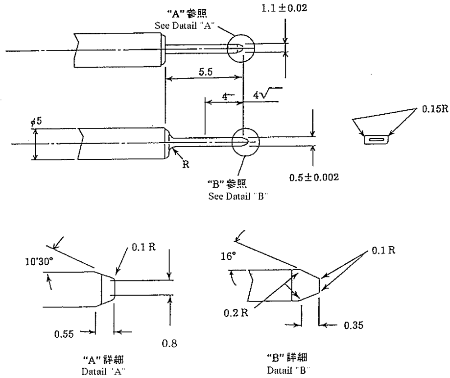
Fig. 10 コンタクト挿入引抜き力測定用ゲージ Fig. 10 Gage Design for Contact Mating/Unmating Force Tests
