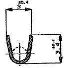
断面 B-B SECT. B-B
