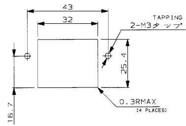
パネル取付寸法 PANEL CUT OUT DIMENSION
