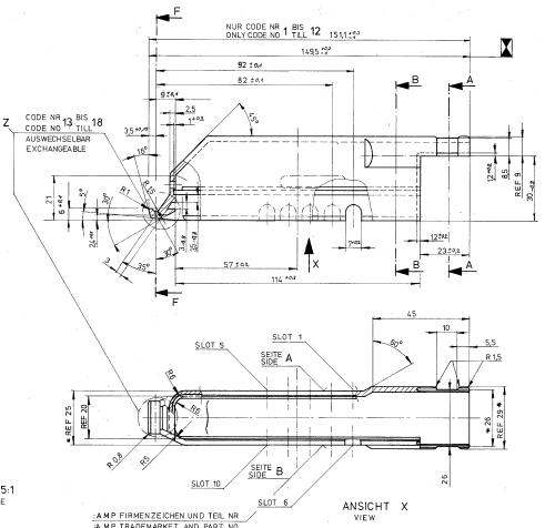
EINZELHEIT Y M 5:1 DETAIL SCALE
