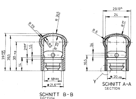
SCHNITT B-B SECTION
