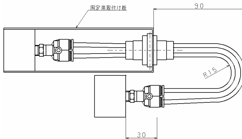
Fig.4 揺動耐久試験
