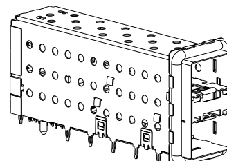
2007538-4 AND 2007538-8 SCALE 3:1
