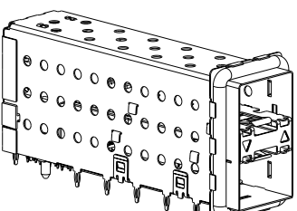
2007538-3 AND 2007538-7 SCALE 3:1
