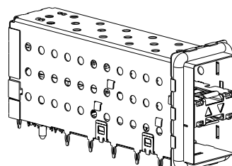
2007538-2 AND 2007538-6 SCALE 3:1
