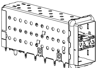
2007538-1 AND 2007538-5 SCALE 3:1
