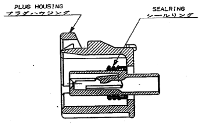
SECT 断面 A-A
