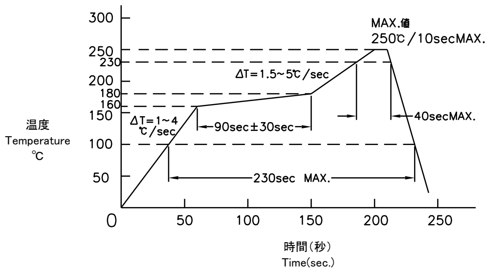
図3 リフロー温度プロファイル Fig.3 Temperature profile of reflow soldering
