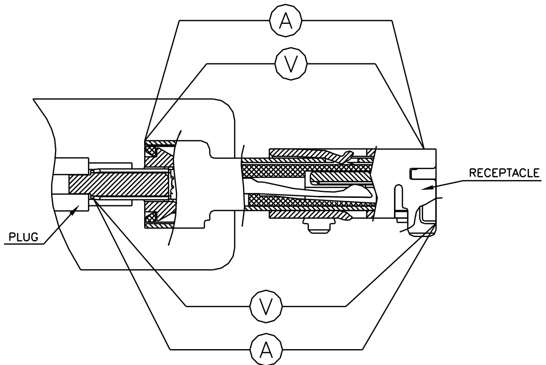
図1 コンタクト及びシェル抵抗測定点 Fig.1 Contact and Shell resistance measuring point
