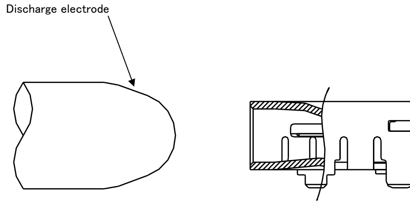
図2 電気放電試験方法 Fig.2 Test method of electrostatic discharge
