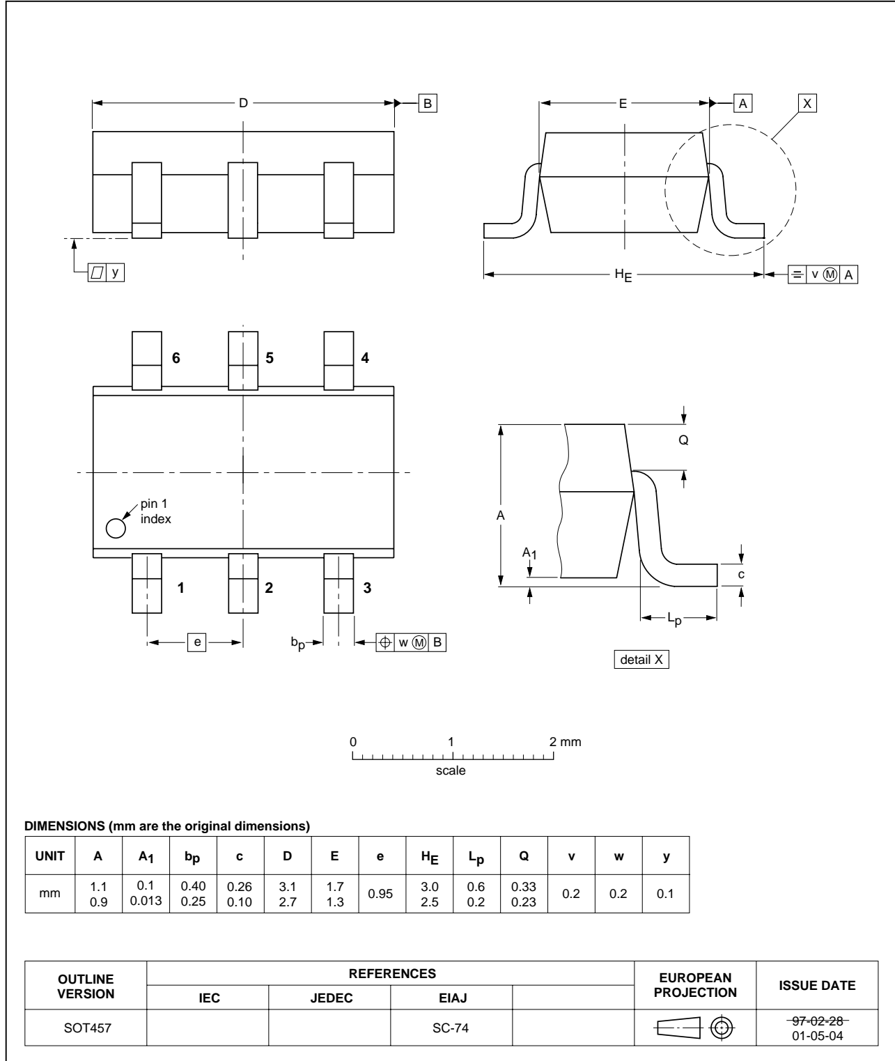
Fig 14. SOT457 (TSOP6).
