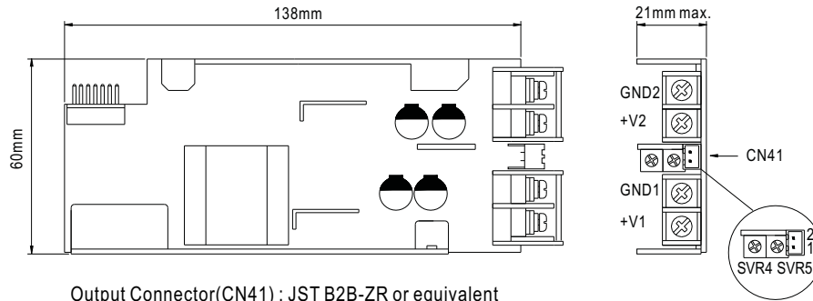
Output Connector(CN41) : JST B2B-ZR or equivalent
