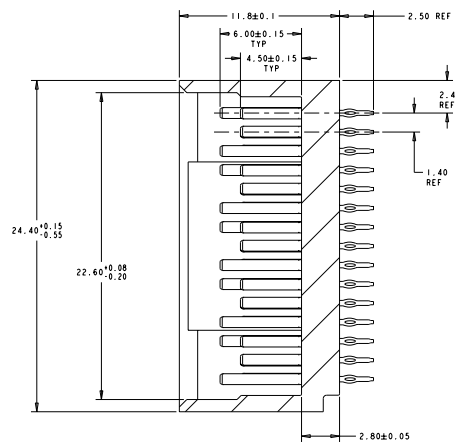
SECTION W - W
