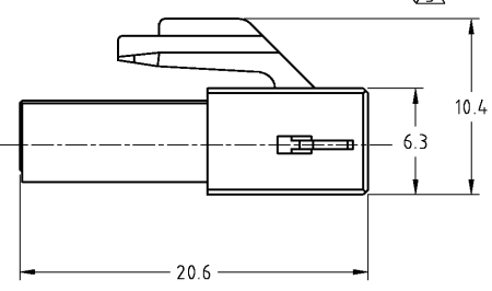
ハウジングロックタイプ A HOUSING LOCK TYPE A
