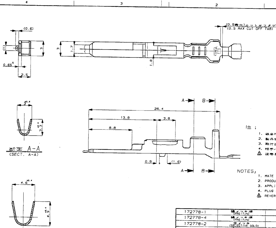
断面 B-B (SECT. B-B)
