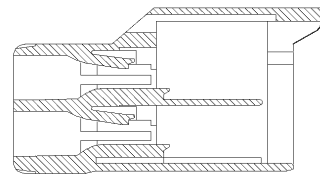
断面A-A
