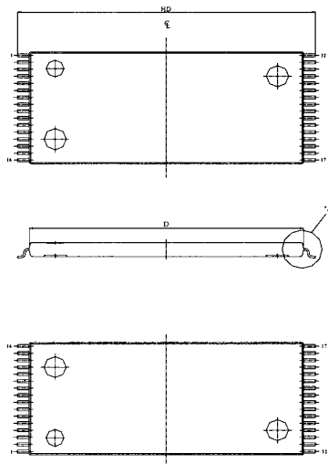
TSOP - 32
