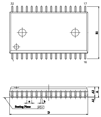
SOP - 32
