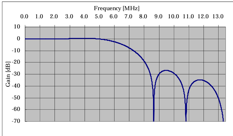
Fig. 3 Chroma-2 LPF
